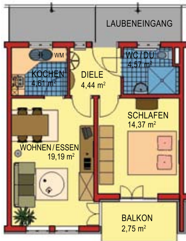
Wohnbeispiel 1: 2-Zimmer, 49,80 qm, Balkon, Einbauküche
